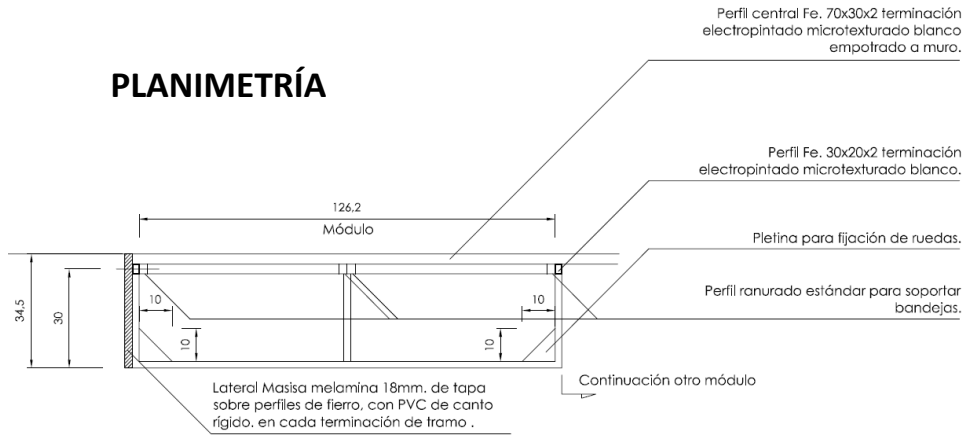
1 PLANTA 1/10
