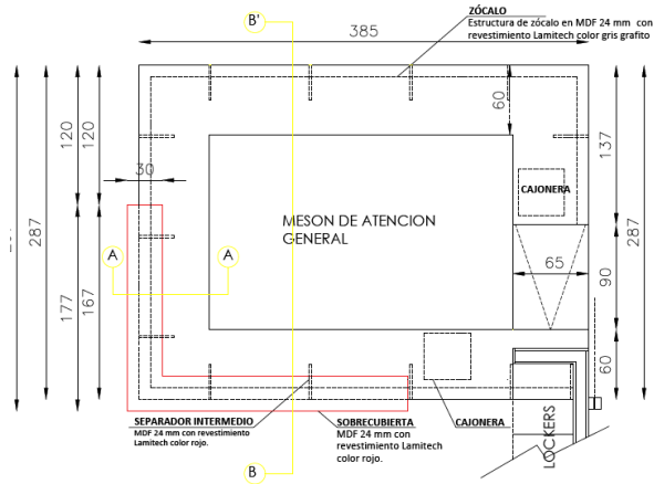
1 PLANTA MESÓN ATENCIÓN
