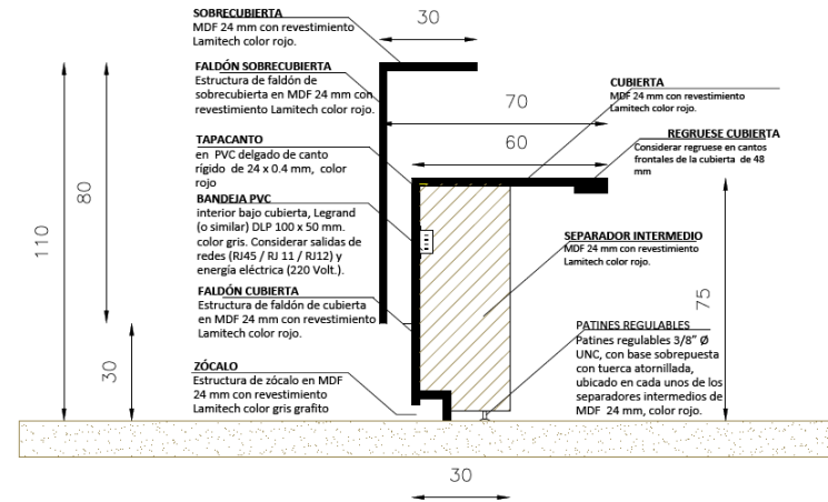
2 CORTE A-A' MESÓN ATENCIÓN
