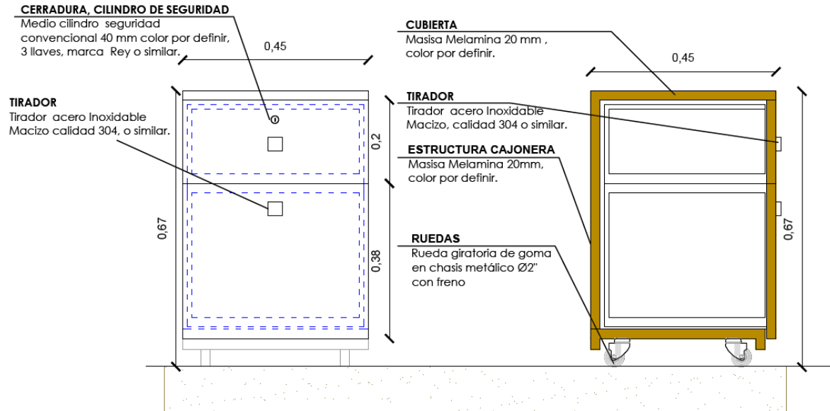
ELEV FRONT- CAJONERA MÓVIL DOBLE CAJON
